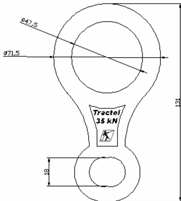
Descendeur 8 de montagne code 20542 8 mountain evacuator code 20542
